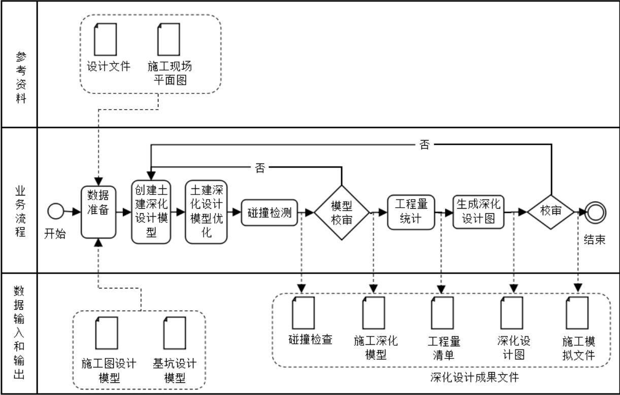
图 5.3.2.1-1 现浇混凝土结构深化设计 BIM 典型应用示意图
