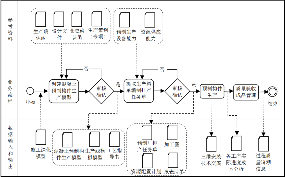
图 5.3.2.2-3 混凝土预制构件生产 BIM 典型应用示意图
