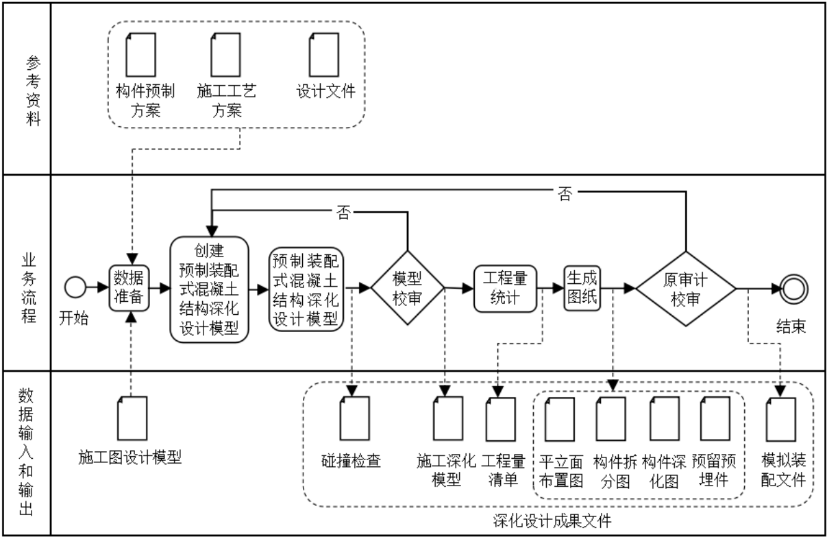
图 5.3.2.1-4 预制装配式混凝土结构深化设计 BIM 典型应用示意图
