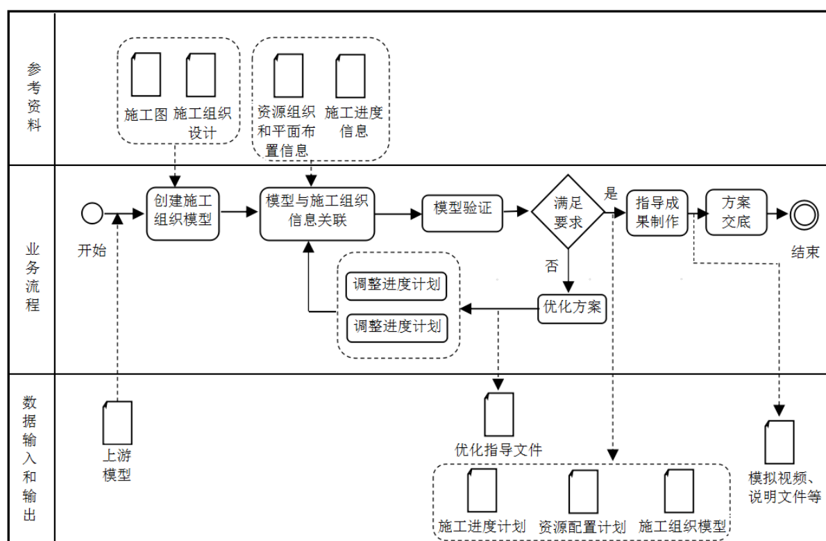
图 5.3.2.7 施工组织模拟 BIM 应用典型流程
