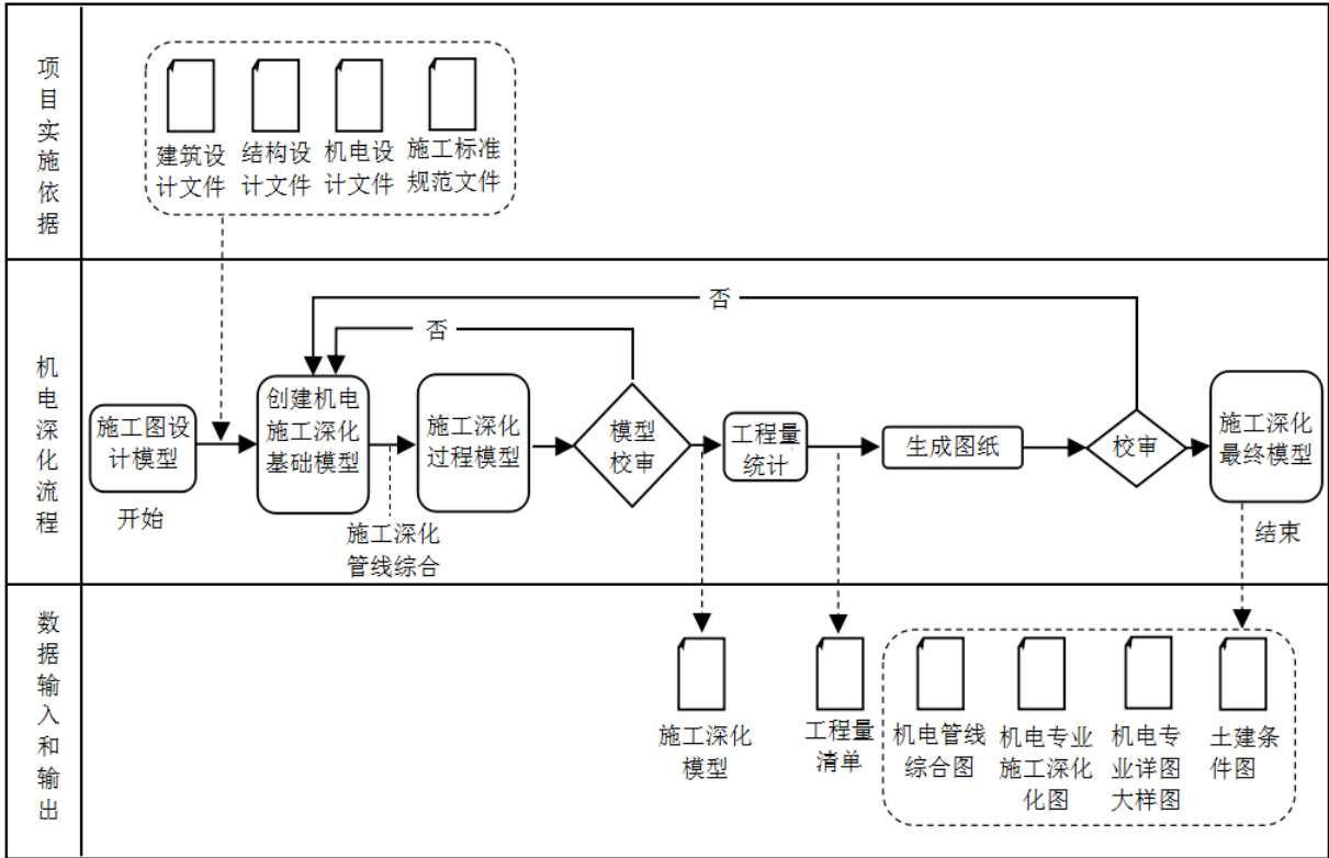
图 5.3.2.1-3 机电施工深化 BIM 典型应用
