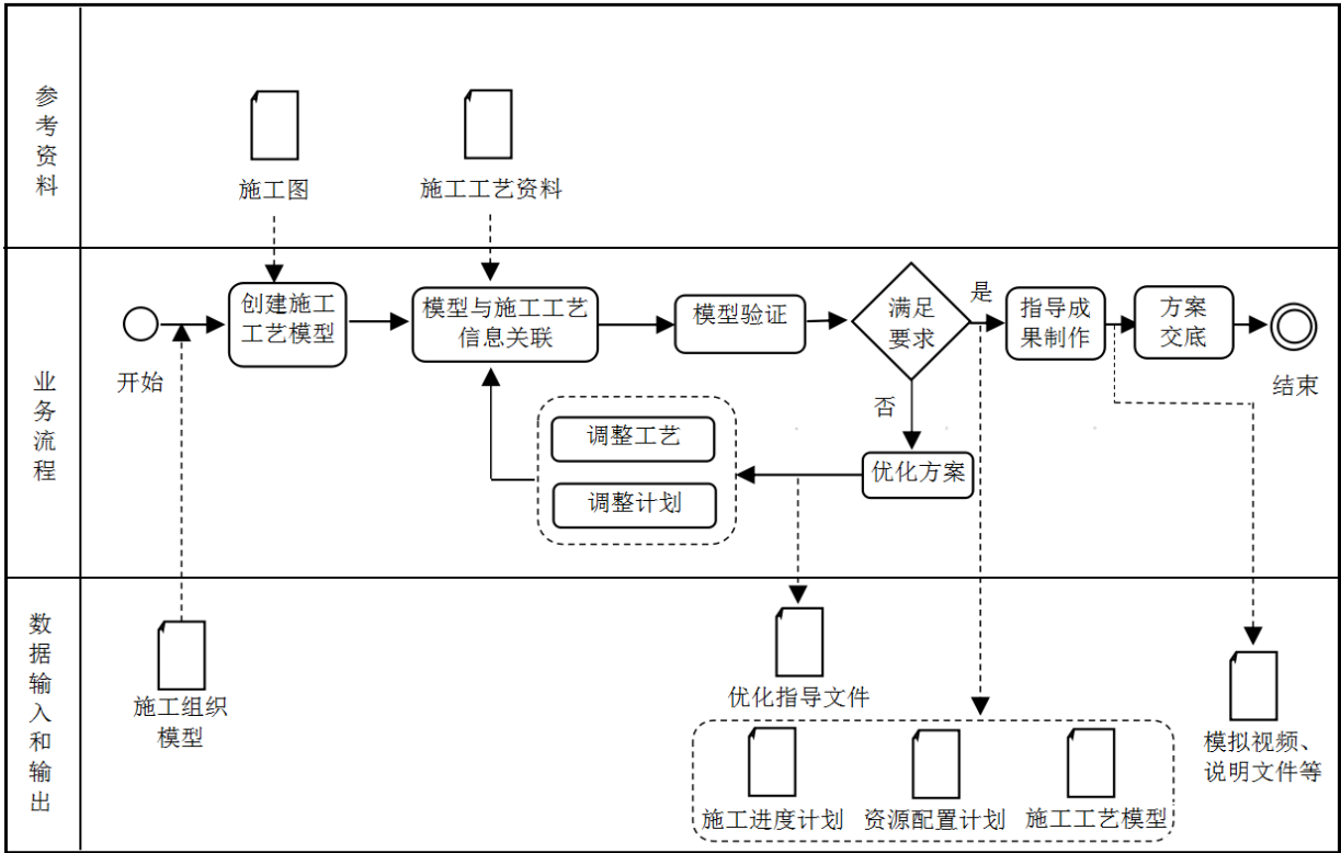
图 5.3.2.8 施工工艺模拟 BIM 应用典型流程
