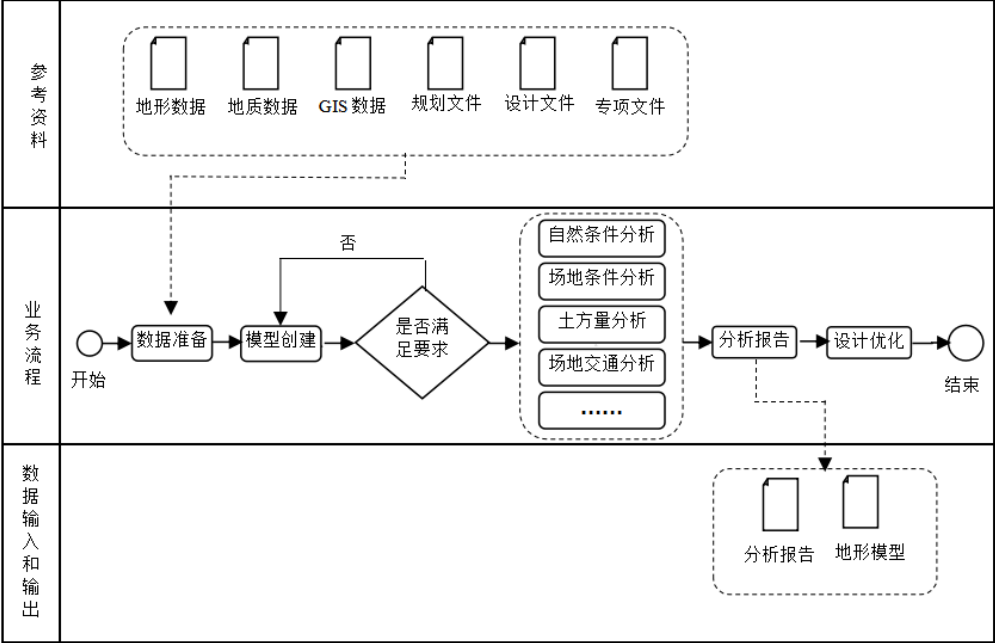
图 5.3.1.1 场地分析 BIM 典型应用示意图
