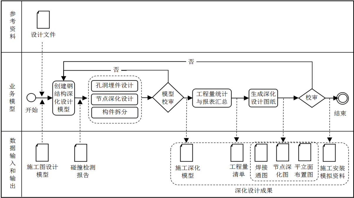
图 5.3.2.1-2 钢结构深化设计 BIM 典型应用
