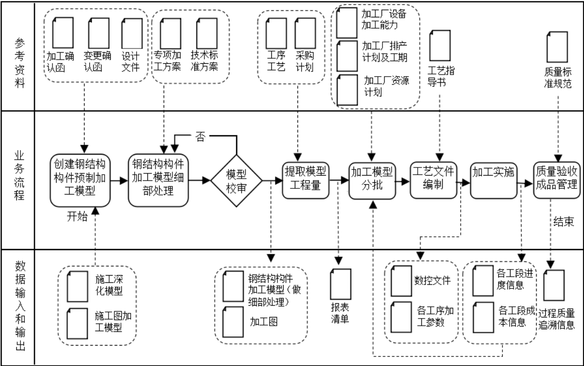
图 5.3.2-1 钢结构构件预制加工 BIM 典型应用示意图
