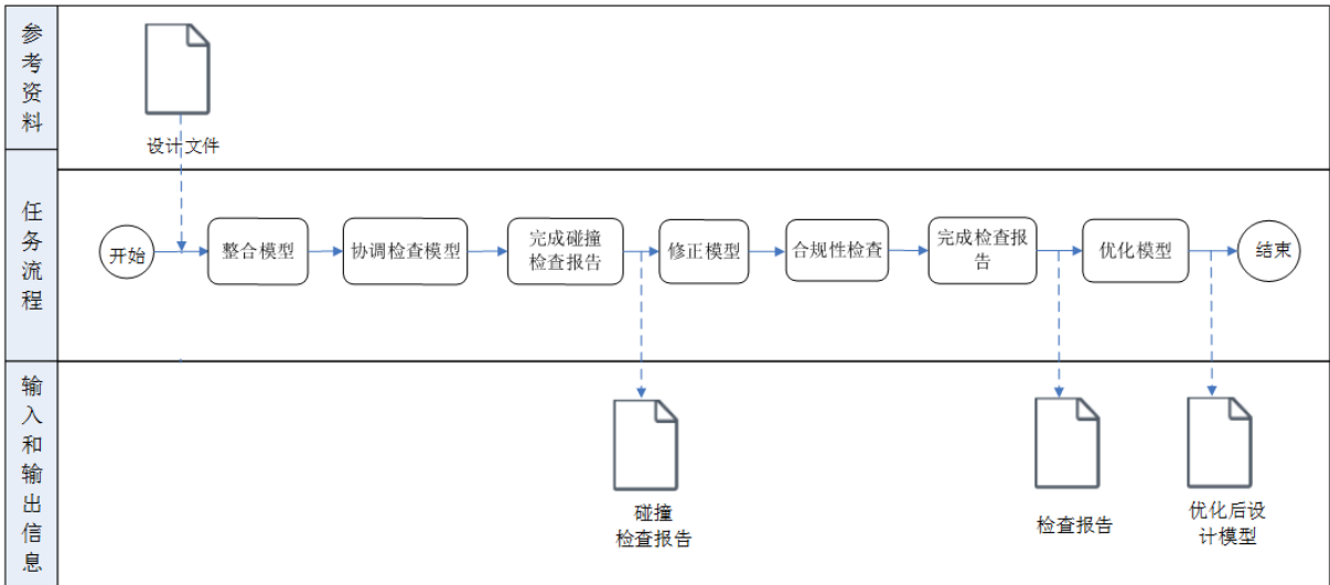
图 5.3.1.7 管综优化 BIM 应用流程
