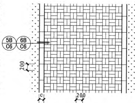
⑫ 烧结砖路面
