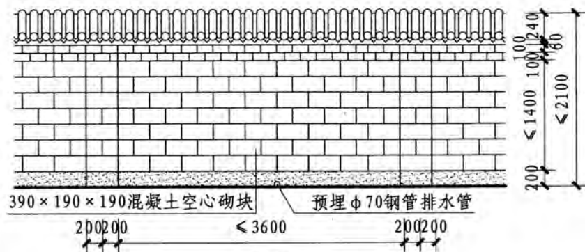
立面
