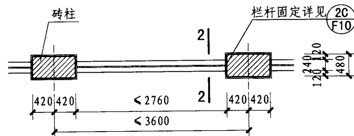
2 砖围墙平面
