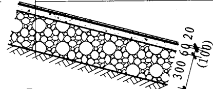
⑥A 水泥豆石抹面坡道(卵石垫层)
