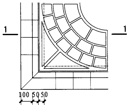
① 带箅子树池平面
