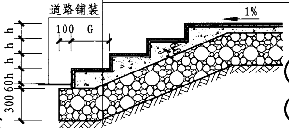
7A 水泥石子剁斧面层台阶 (卵石垫层)
