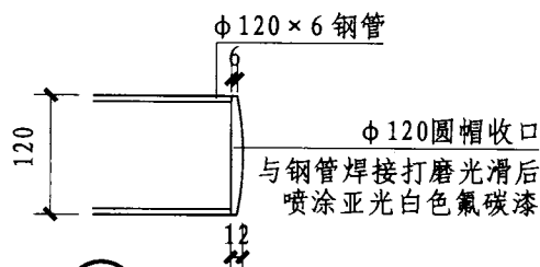
(c) 钢管收口大样二
