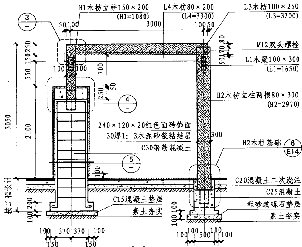
③ 木柱连接详图
