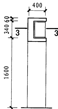
② 门柱灯立面
