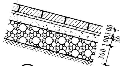
12A 花岗岩面层坡道(卵石垫层)
