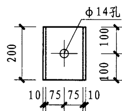
钢套一侧视图
