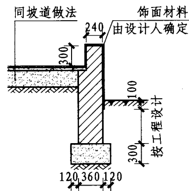
E 坡道侧挡墙做法
