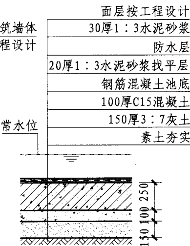
B2 池底内防水做法
