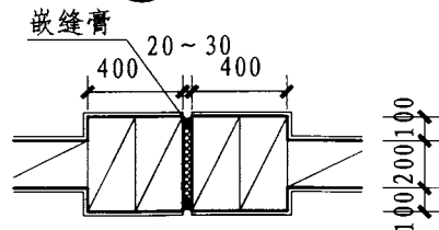
d 混凝土砌块墙变形缝
