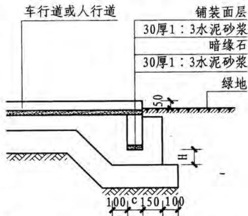
8A 混凝土暗缘石 8B 石材暗缘石
