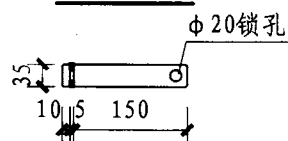
插销平面
