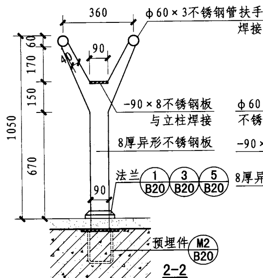
2B 钢管中间扶手
