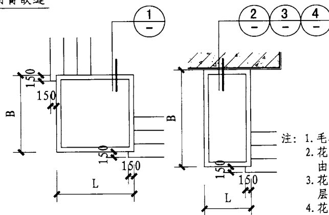
花池平面位置示意图
