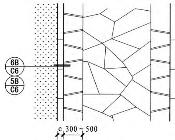
③ 碎石板与花岗岩路面
