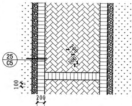
⑪ 水泥砖与散置卵石路面
