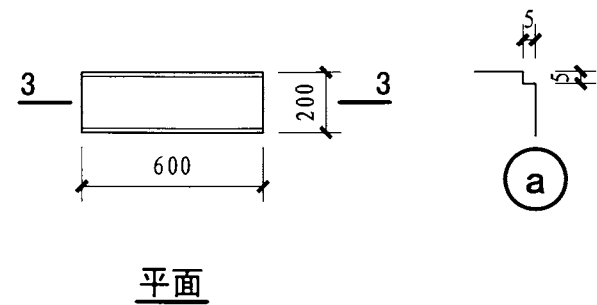
③ 花岗岩卧式路障
