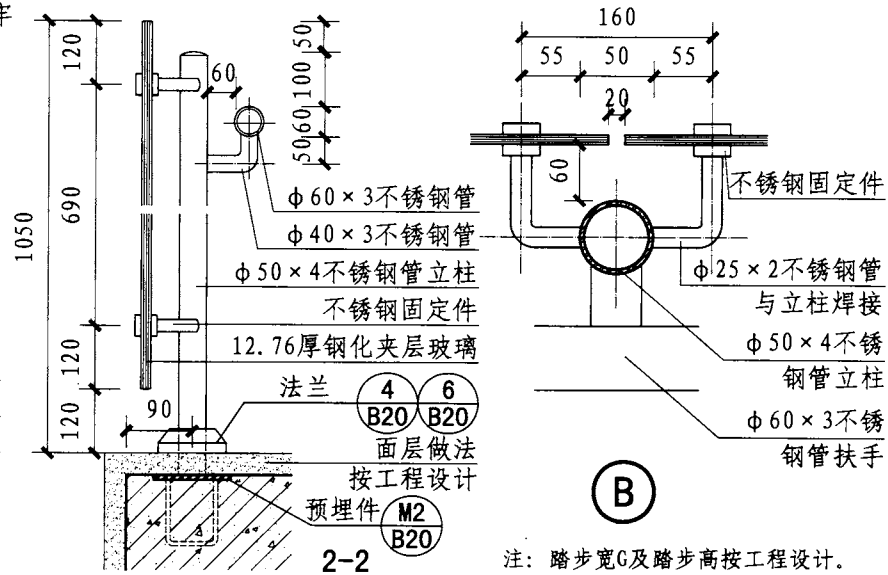
玻璃栏板
