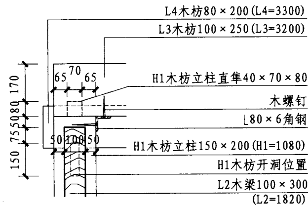
③ 木柱连接详图
