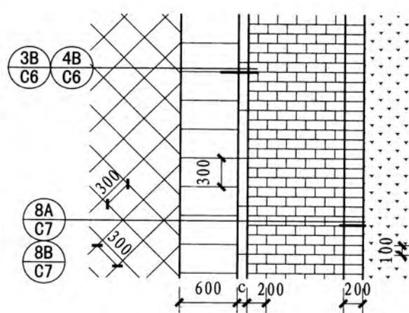
⑬ 花岗岩透水砖路面
