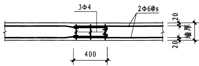
墙体水平拉结筋连接详图
