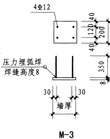
框架梁(板)预埋件
