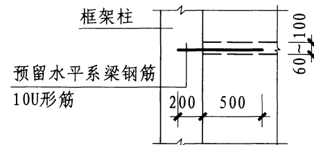
预留水平系梁钢筋
