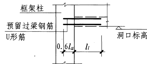
柱边洞口预留过梁钢筋
