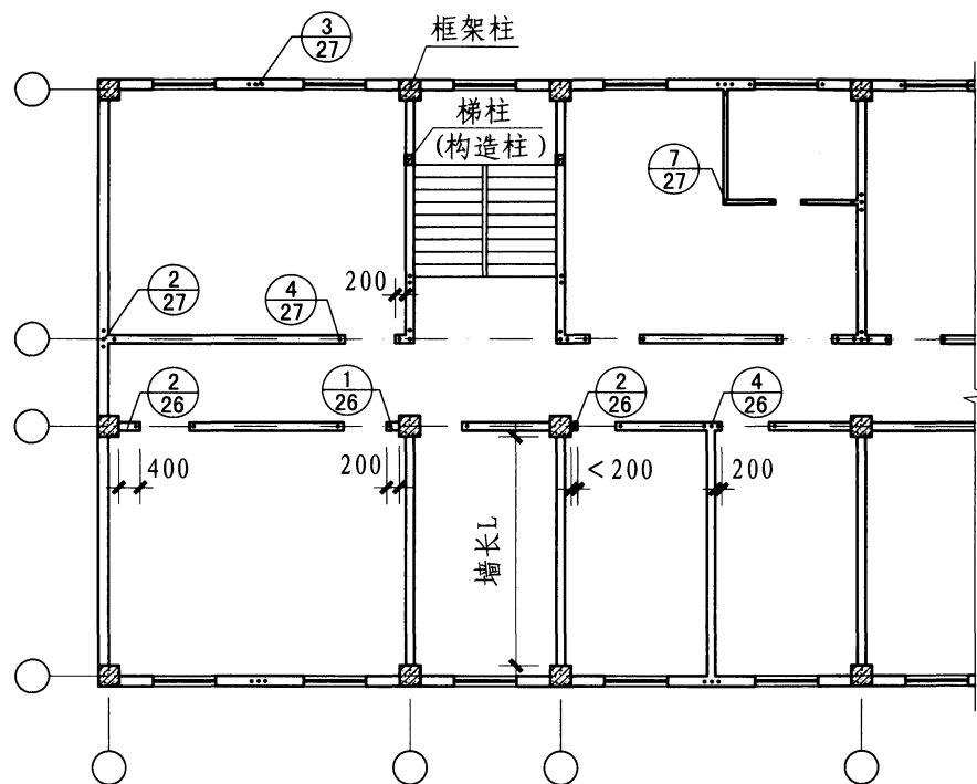
小砌块填充墙芯柱布置平面示意图
