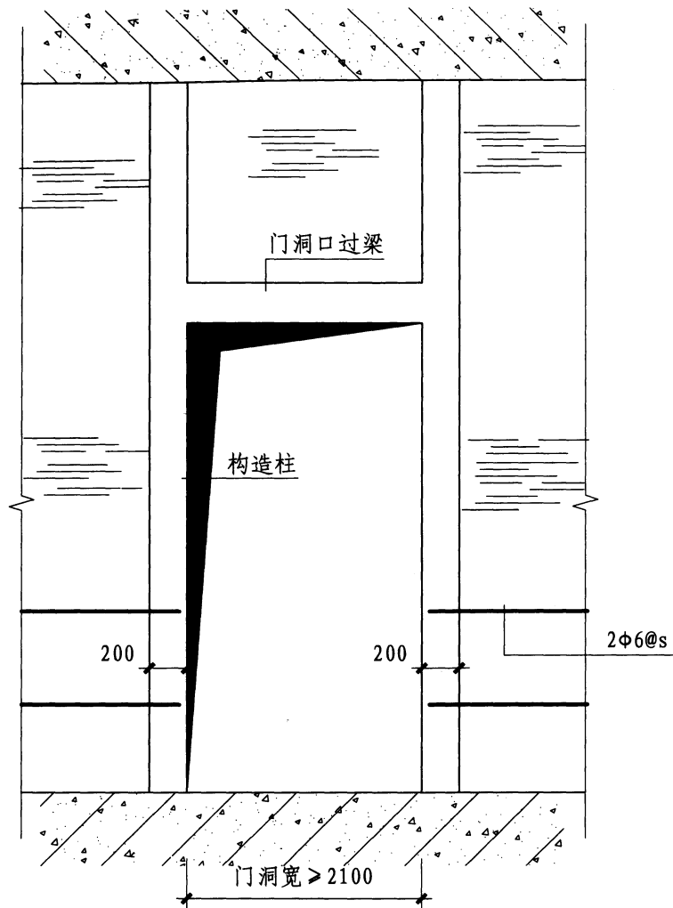
门洞口做法(二)
