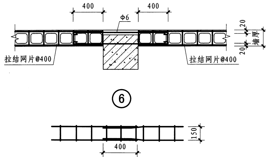
拉结网片搭接连接详图
