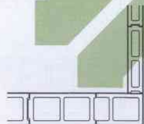
②a 190厚与90厚墙转角处偶数皮平面
