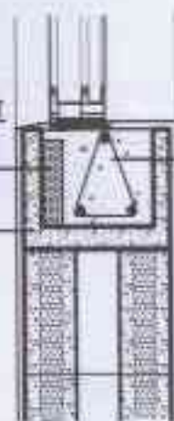
② 窗台处设通 长水平系梁
