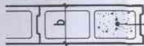
① 门洞边砌块灌芯柱 90厚砌块墙不设芯柱
