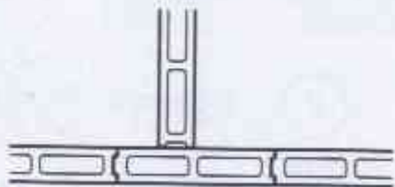
③a 90厚墙丁字交接 奇数皮平面
