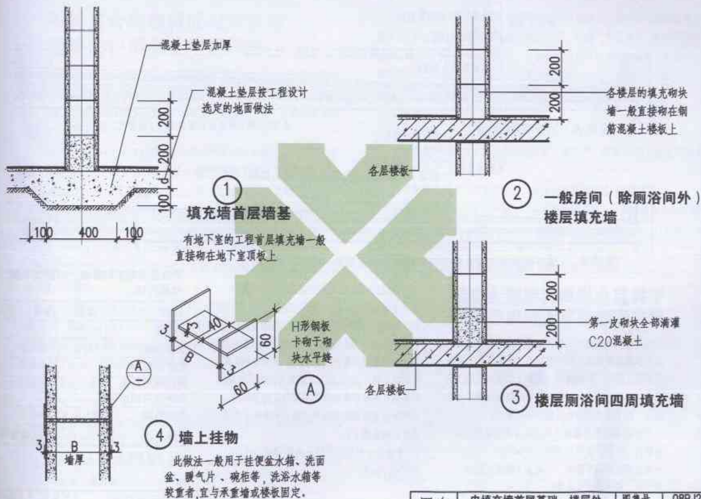
图名 内填充墙首层基础、楼层处填充砌块墙砌筑、墙上挂物
