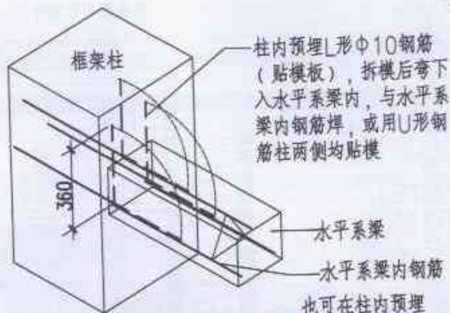
① 框架柱内预埋贴皮钢筋 也可在柱内预埋 6X200X200 钢板, 水平系梁内钢筋与钢板焊接
