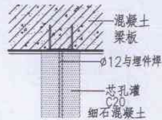
(A) 芯柱插筋与梁板连接
