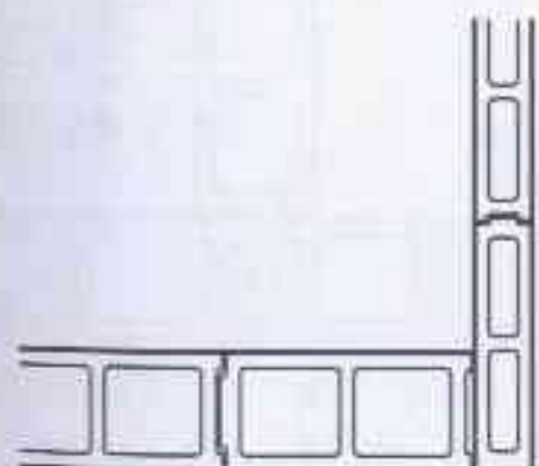
② 190厚与90厚墙转角处奇数皮平面
