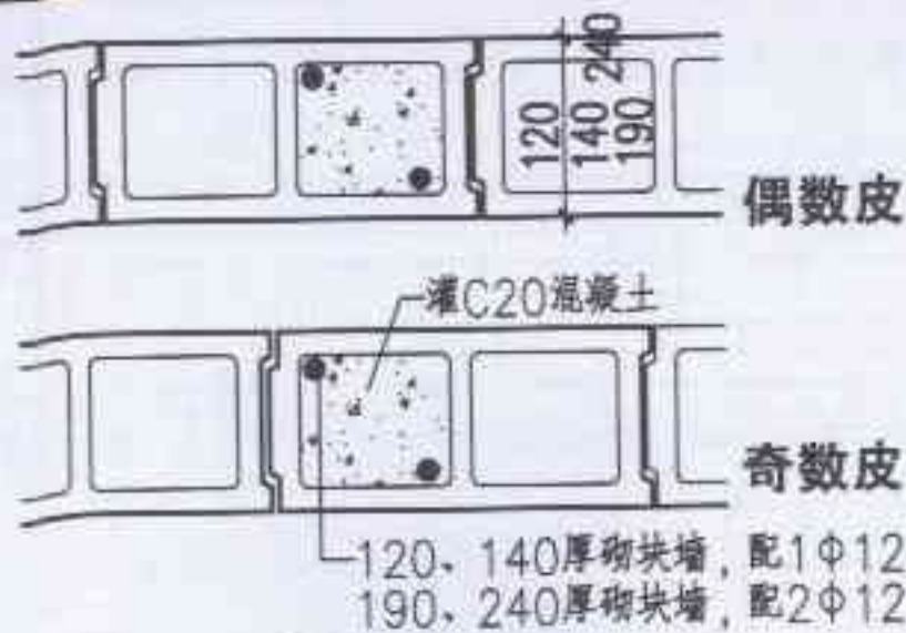
④ 芯柱
