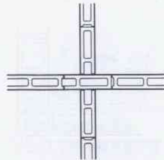
②a 90厚墙十字交接 奇数皮平面
