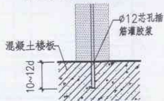
③ 芯柱插筋与楼板连接
