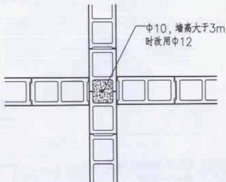
③ 190厚墙十字交接 奇数皮平面
