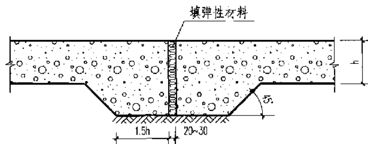
④ 伸缩缝 20 ~ 30m
