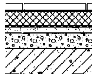
发泡聚氨酯上人屋面 倒置式
