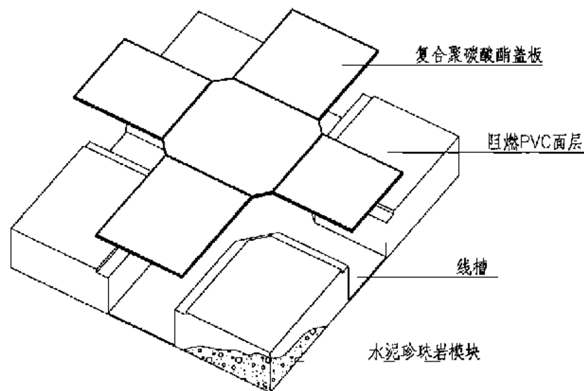
平铺型网络地板结构示意
