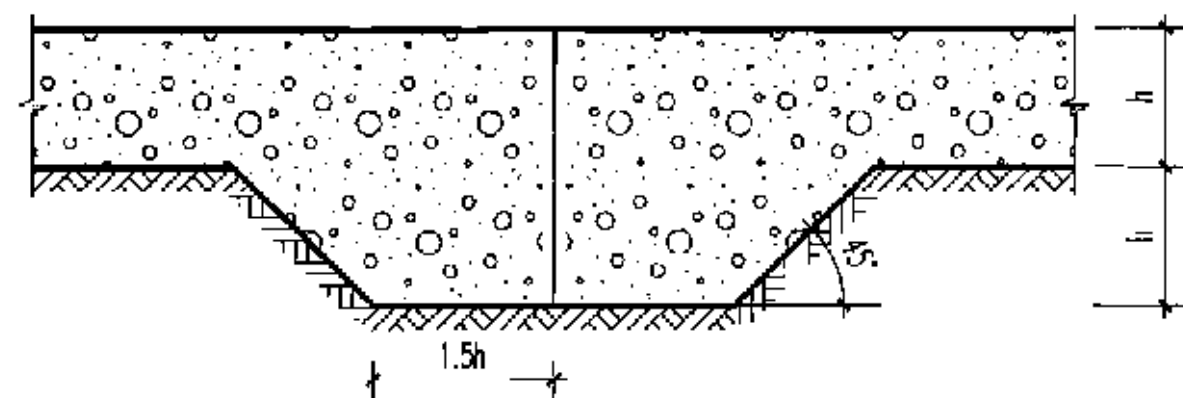
⑤ 垫层分仓周边加肋缩缝 6 ~ 12m
