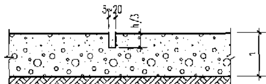
③ 横向缩缝 6 ~ 12m
