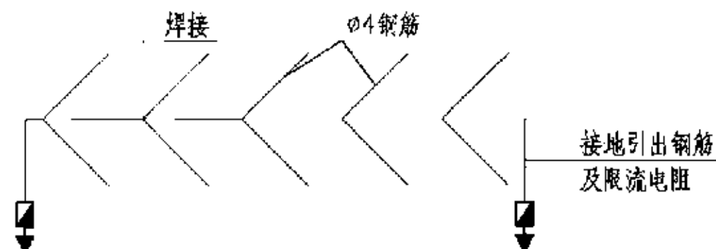
鱼骨状导静电接地网
