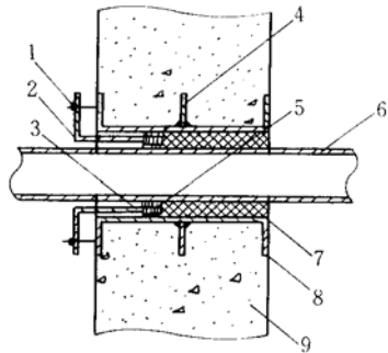
图 9.5.2—2 套管式穿墙管构造图
