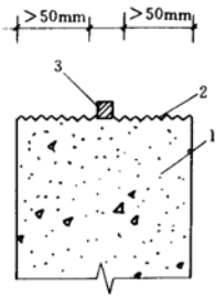
图 9.2.10—1 遇水膨胀胶条 安装断面图 1—主体结构；2—施工缝；3—膨胀胶条 注：膨胀胶条应采取防过早膨胀措施 并粘贴牢固。 图 9.2.10-2 遇水膨胀胶条 搭接平面图 1—主体结构；2—膨胀胶条 注：膨胀胶条应采取防过早膨胀措施 并粘贴牢固。
