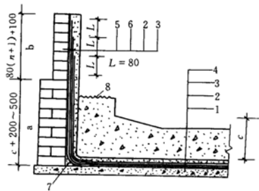
图 5.8.1 先贴防水层卷材铺贴图
