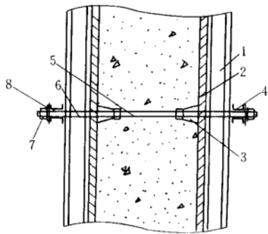
图 5.6.3 模板拉杆螺栓连接图
