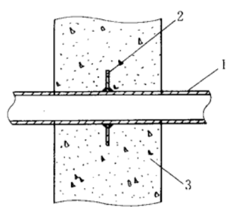
图 9.5.2—1 穿墙管图
