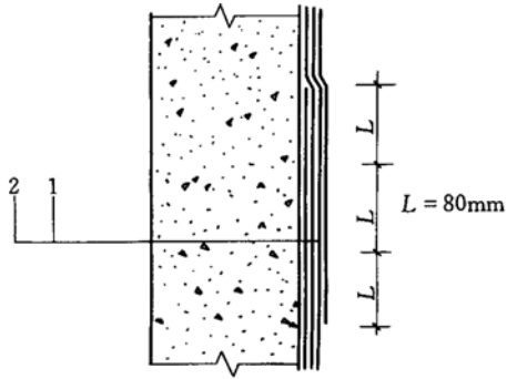
图 5.8.2 卷材错茬相接构造图
