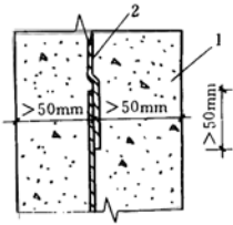
图 9.2.10—1 遇水膨胀胶条 安装断面图 1—主体结构；2—施工缝；3—膨胀胶条 注：膨胀胶条应采取防过早膨胀措施 并粘贴牢固。 图 9.2.10-2 遇水膨胀胶条 搭接平面图 1—主体结构；2—膨胀胶条 注：膨胀胶条应采取防过早膨胀措施 并粘贴牢固。
