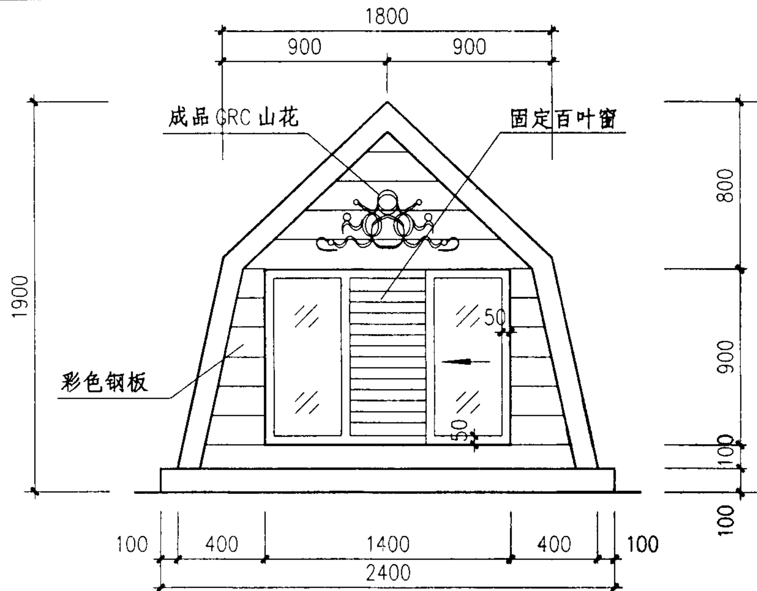
立面
