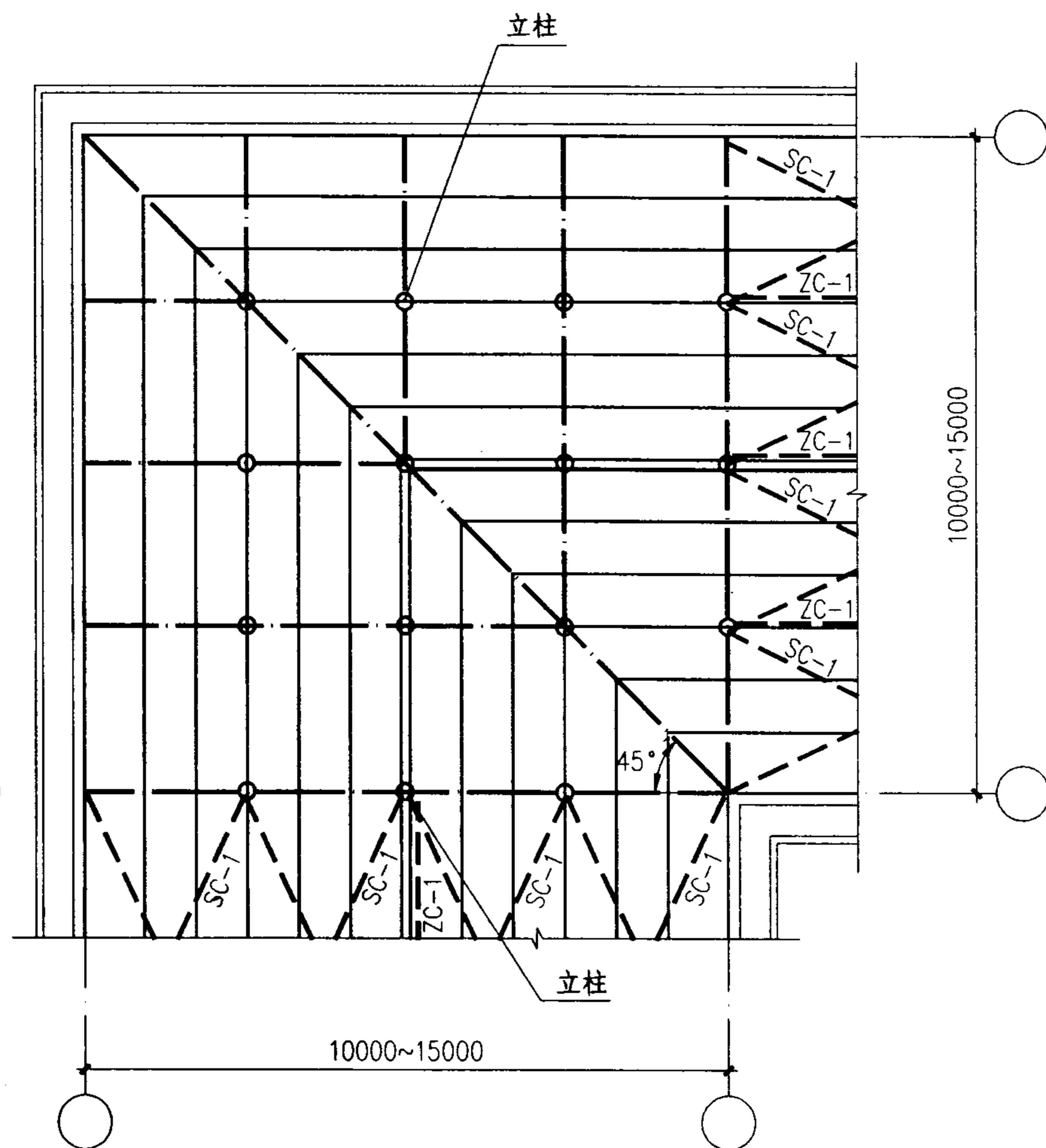
PB-7a PB-7b 屋面钢结构布置图 PB-7c
