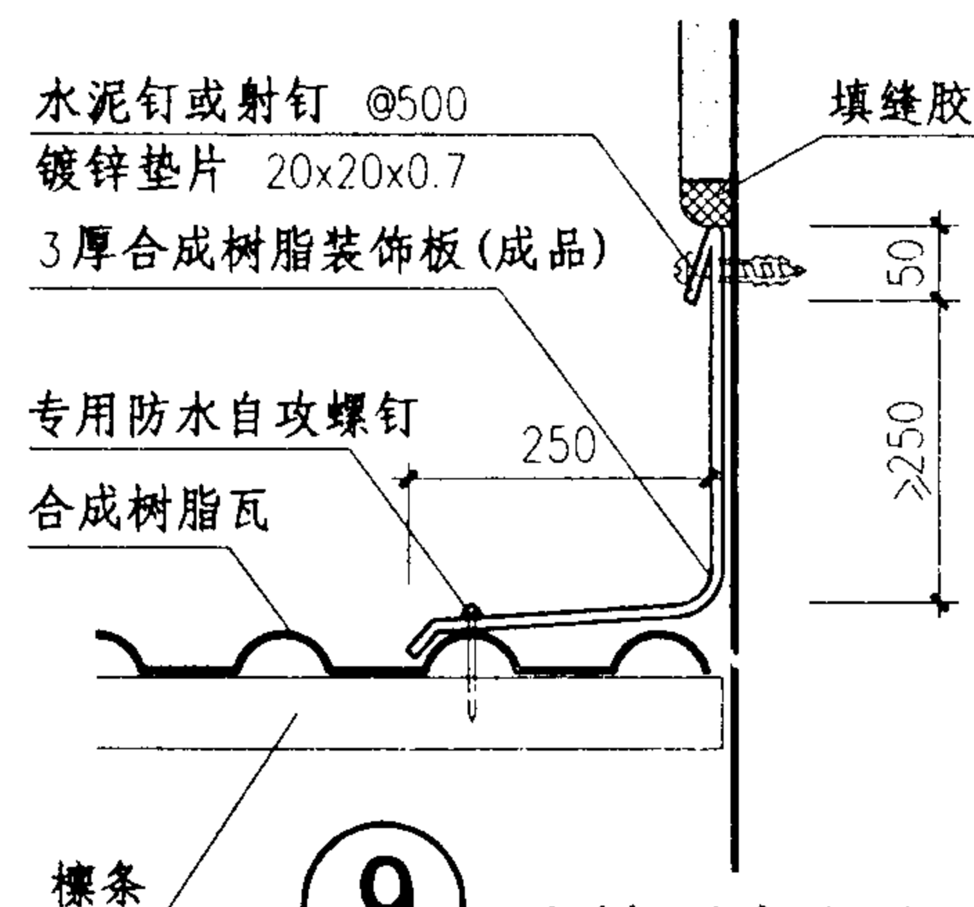
立墙泛水(三)
