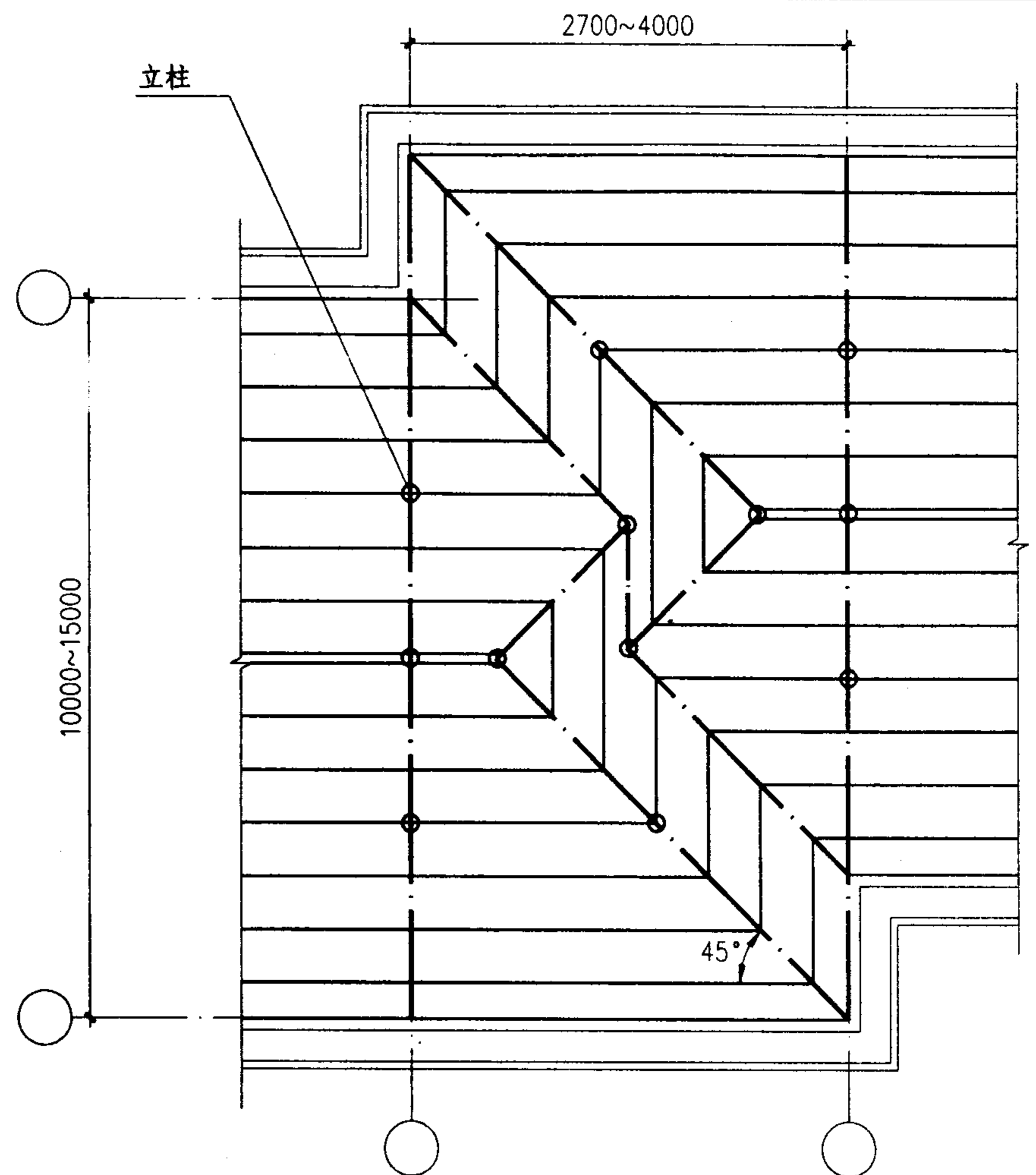
PB-5a PB-5b 屋面钢结构布置图 PB-5c
