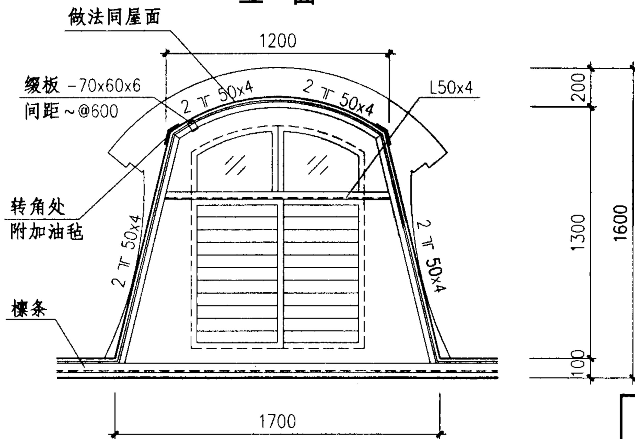
横向剖面
