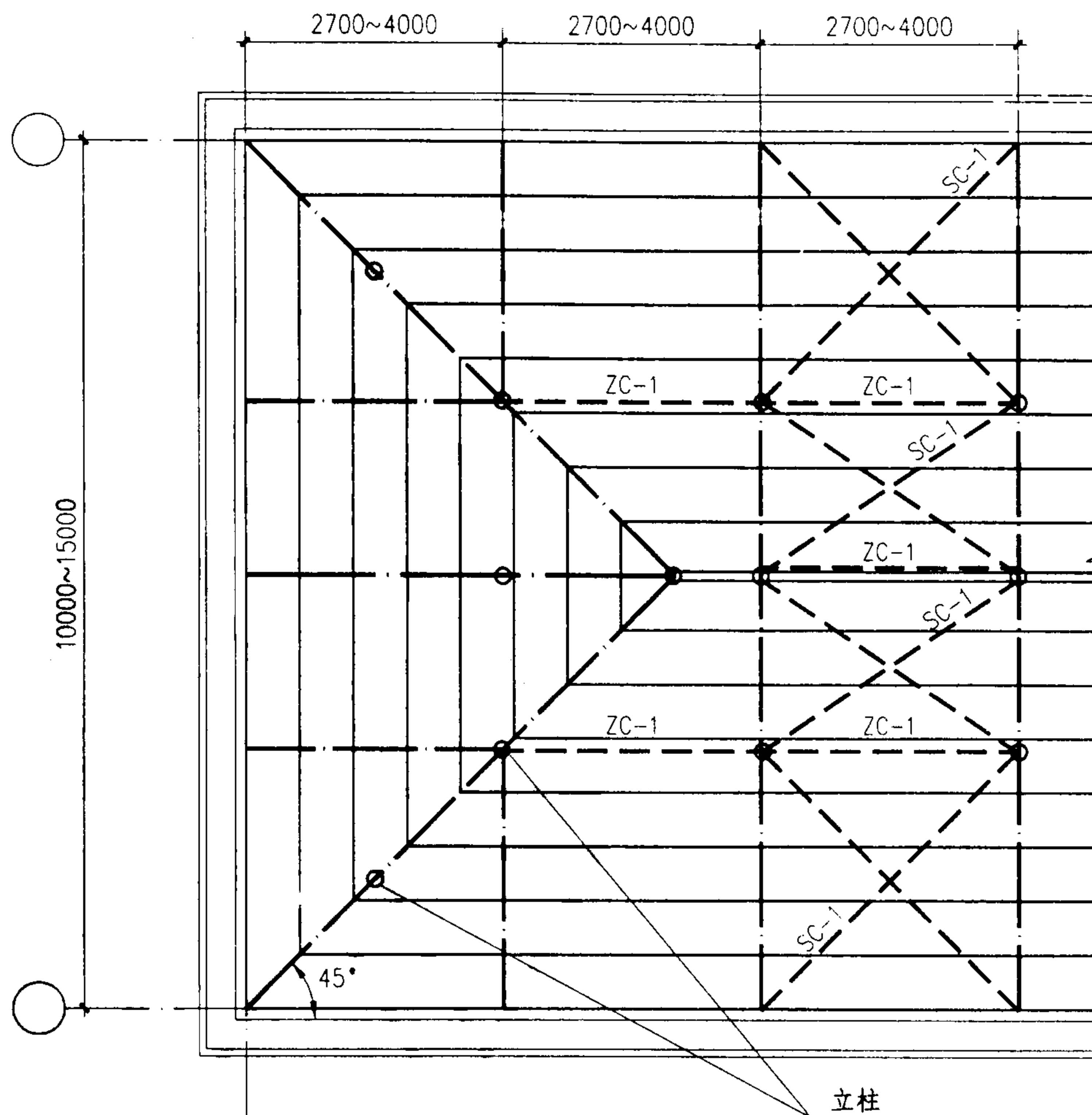
PA-3a PA-3b 屋面钢结构布置图 PA-3c
