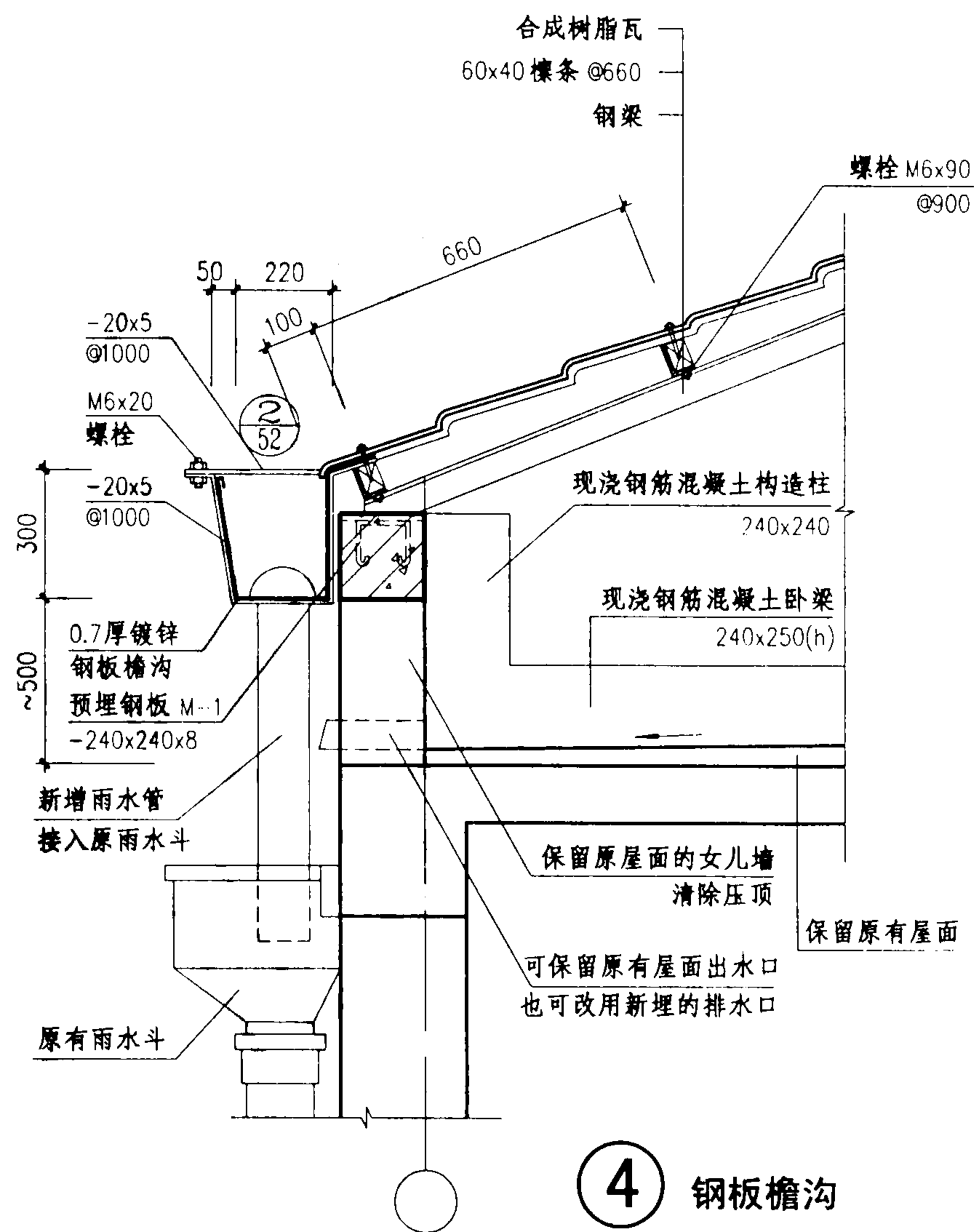
合成树脂瓦屋面檐口详图(二)
