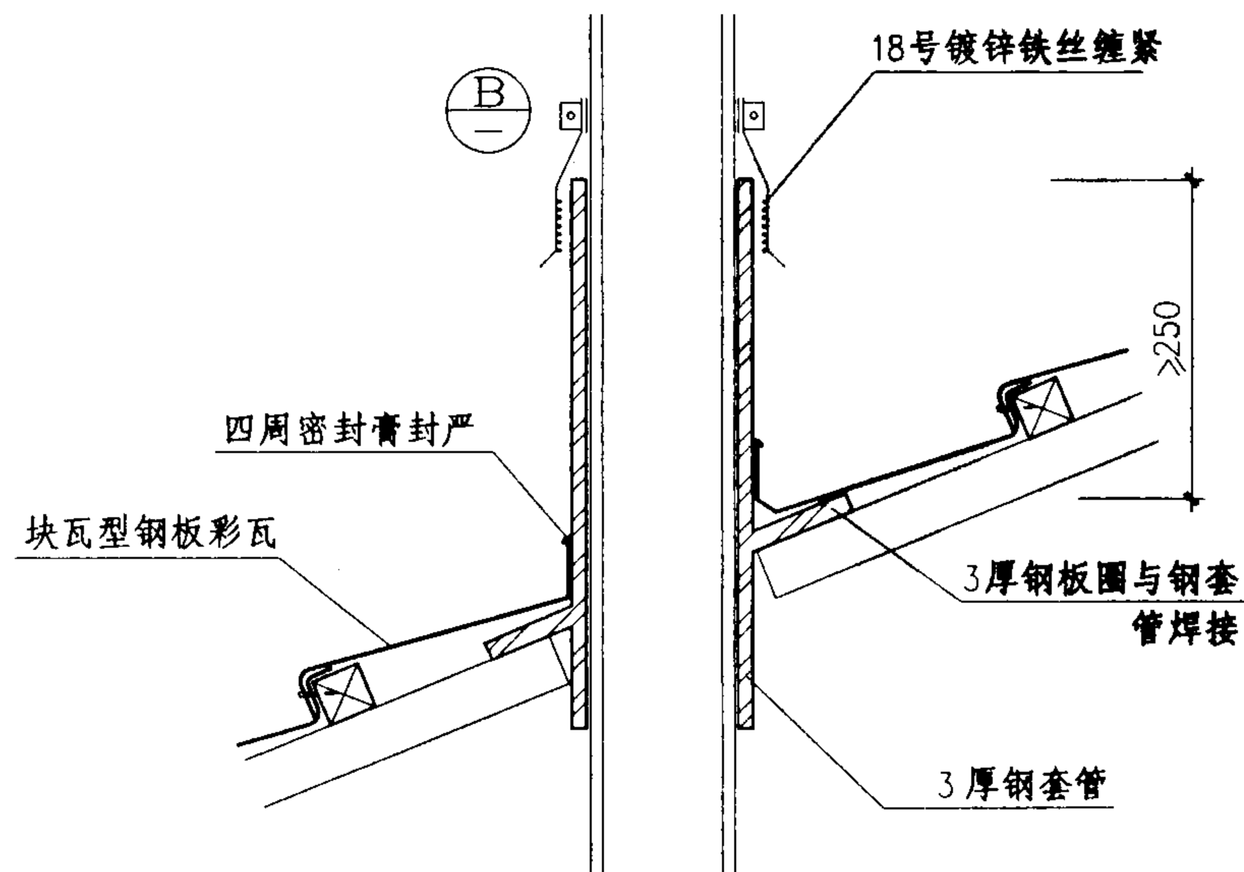
⑩ 管道出屋面泛水
