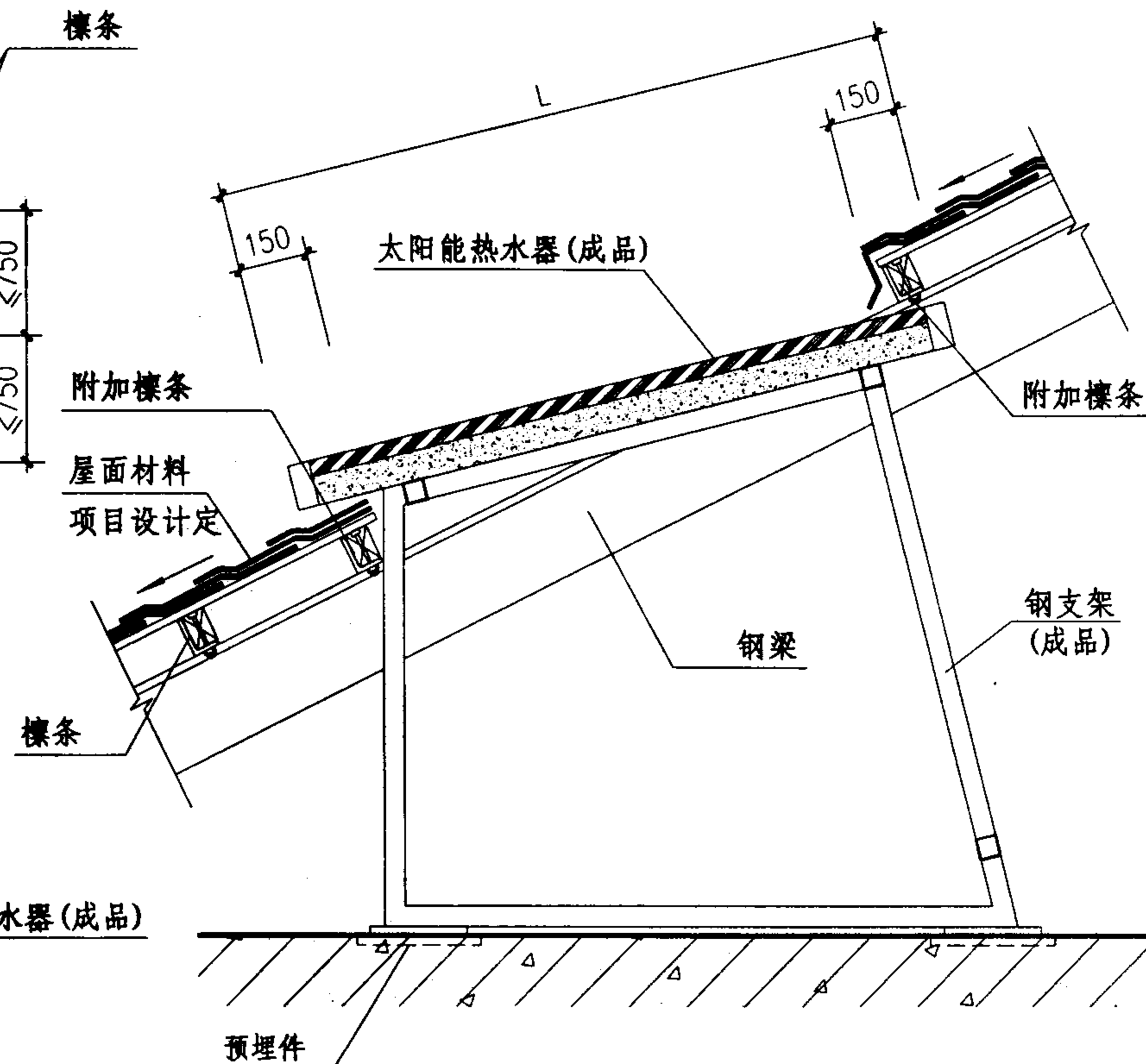
1—1 (支架式放在原有屋面上)
