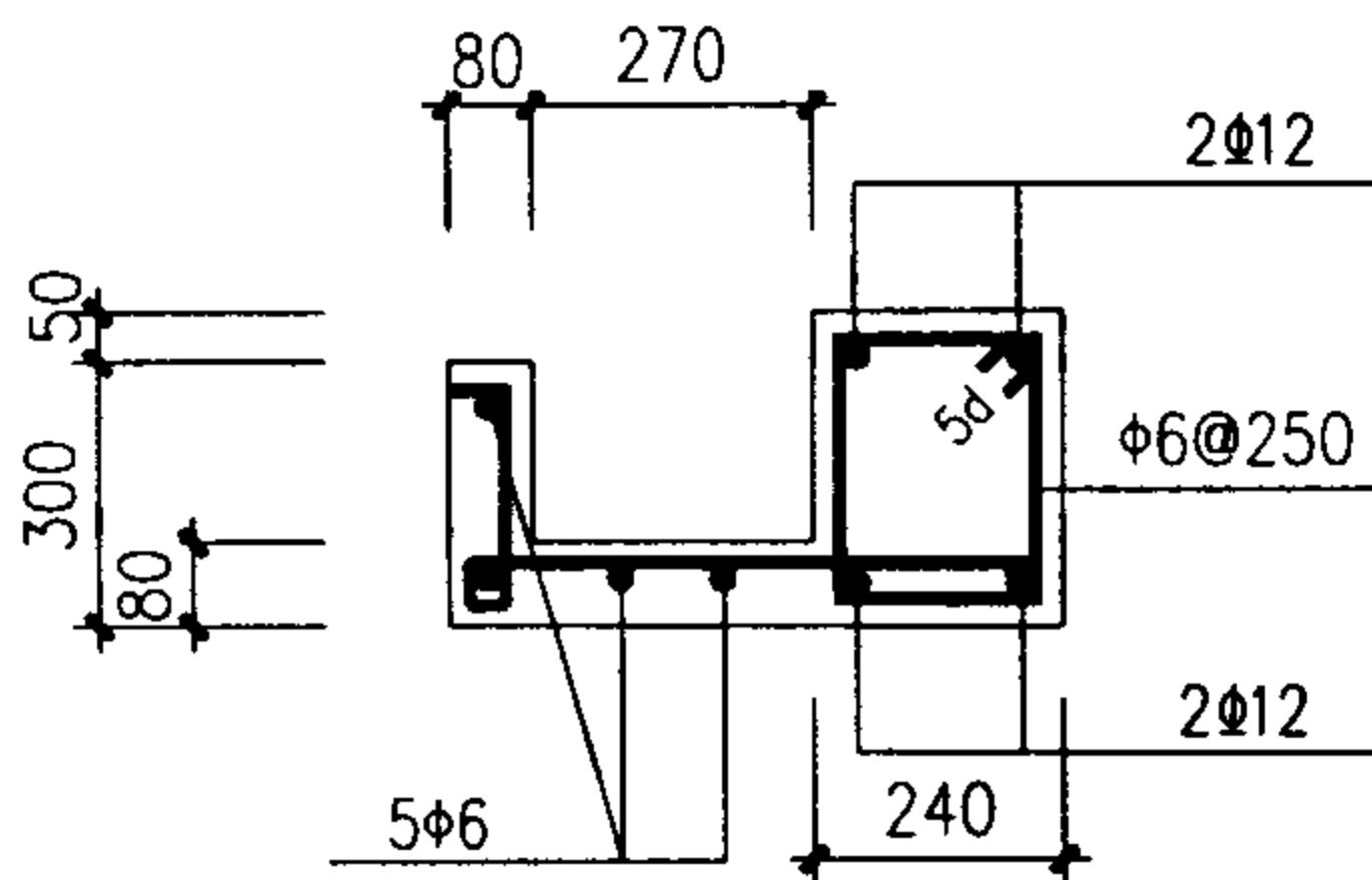
天沟大样(二)
