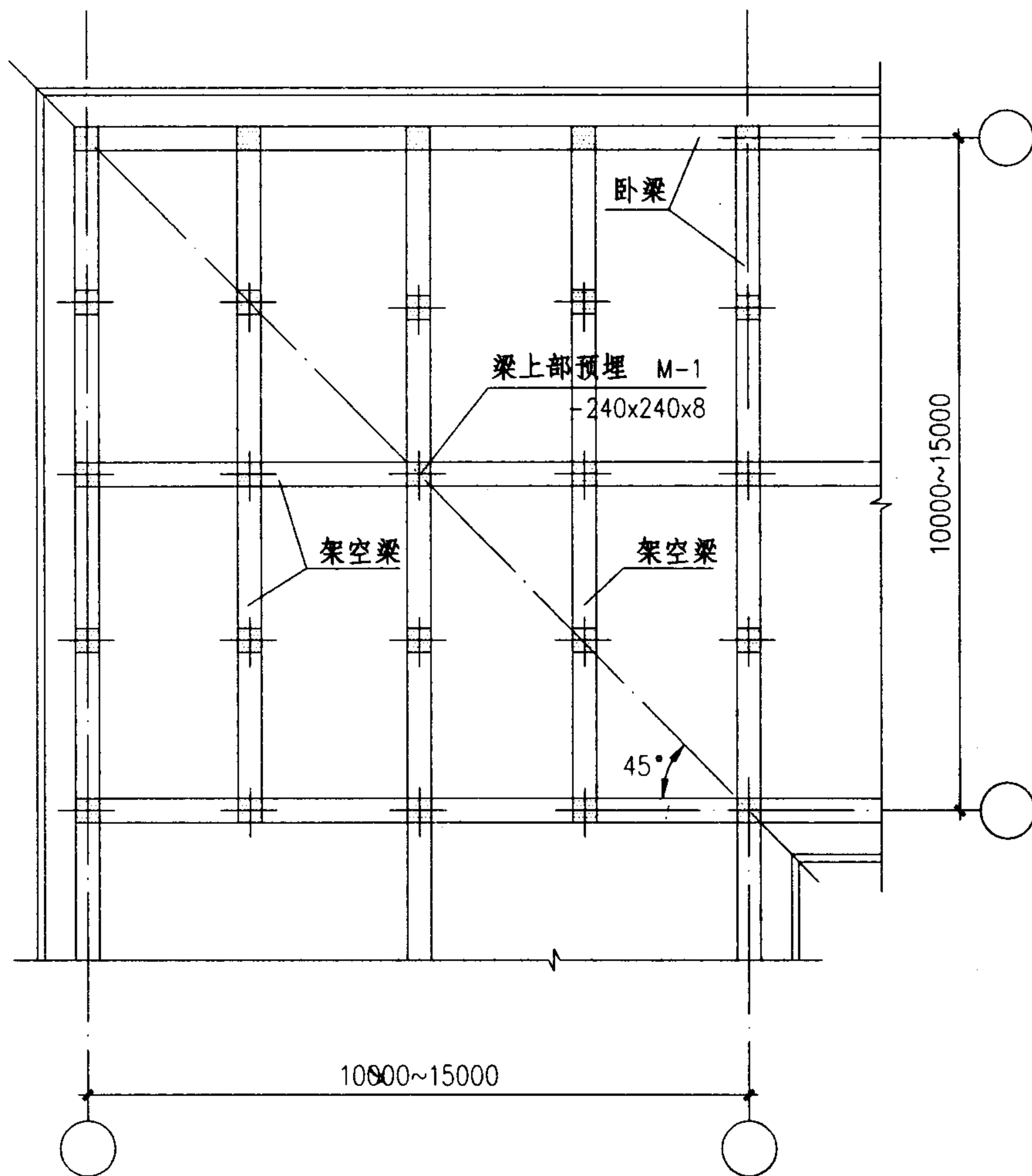
PB-7a PB-7b 屋顶卧梁布置图 PB-7c
