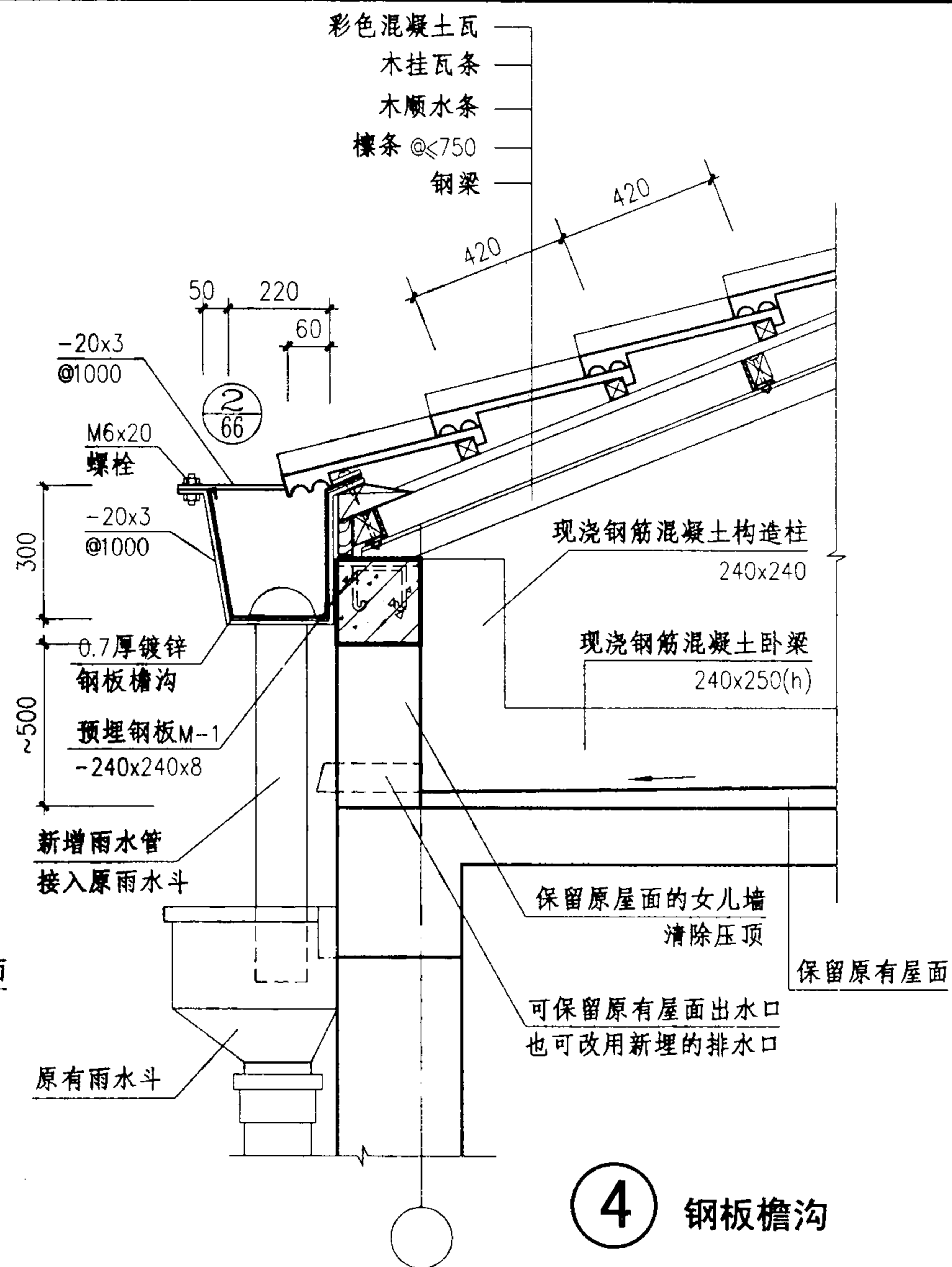
彩色混凝土瓦屋面檐口详图(二)
